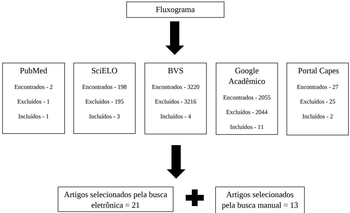
Figura 1 - Fluxograma
