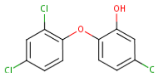
FIGURA 8: Molécula química do triclosan. Fonte: https://pt.wikipedia.org/wiki/Triclosan
