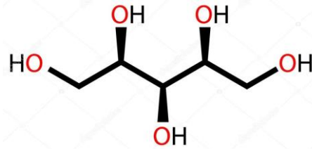
FIGURA 15: Composição química do xilitol. Fonte:
