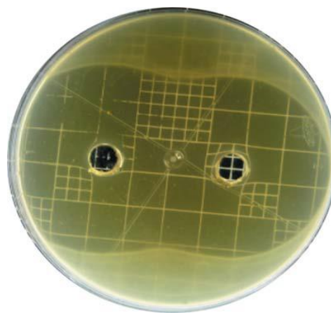
FIG. 2. Inibição de crescimento do Streptococcus mutans utilizando o peróxido de hidrogênio a 1,5%. Fonte: MOREIRA et al. , 2009 pág. 157
